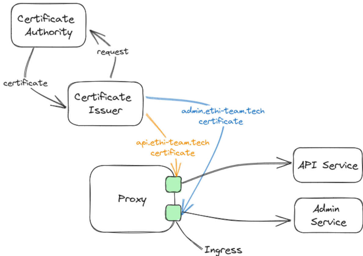
Hình 3.34: Mô hình phân phối tín chỉ TLS
